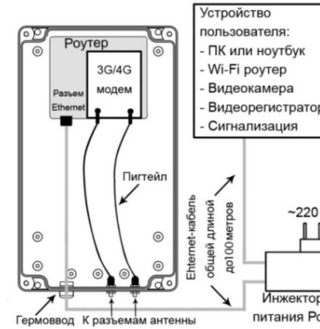
Пример размещения оборудования в гермобоксе
