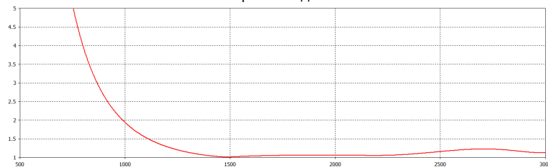
КСВ антенны в рабочем диапазоне частот
