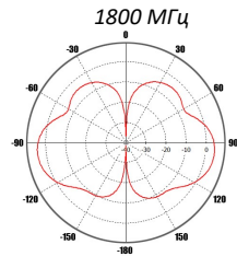
Диаграммы направленности антенны в рабочем диапазоне частот
